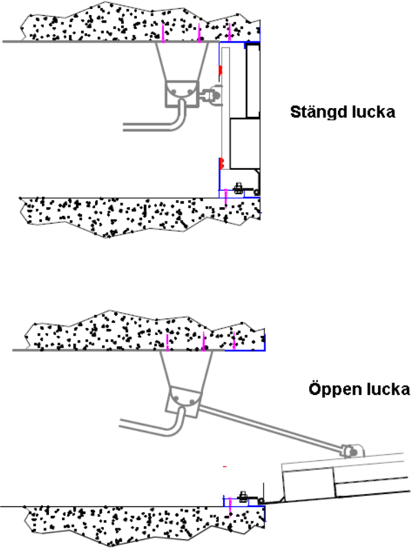
Genomskärningsritning
