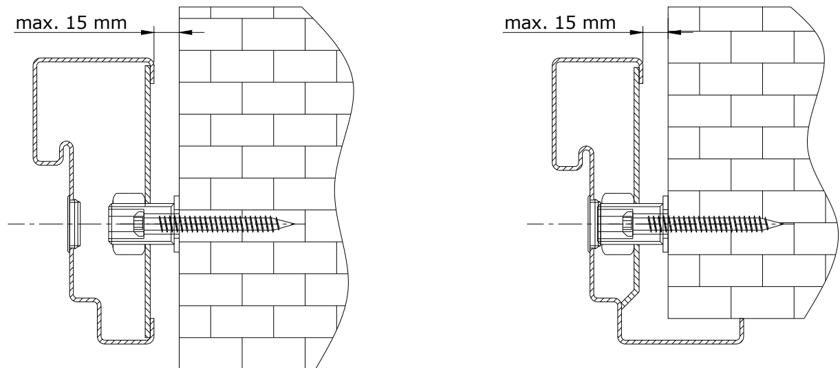
Figur 2. Infästning av en ram med hylsor
