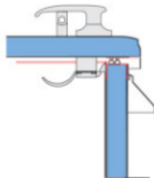
Snabblås samt förberedd för hänglås på utsidan
